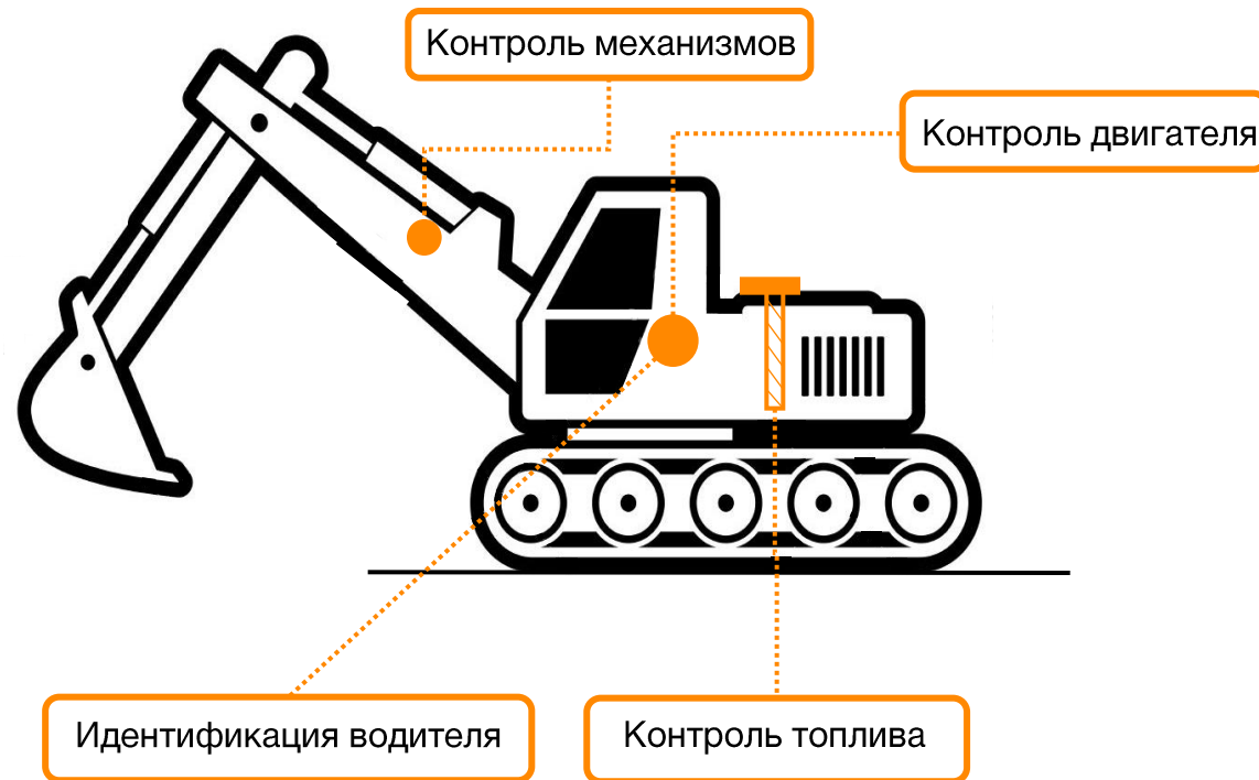
Варианты фиксации датчиков на механизмы
